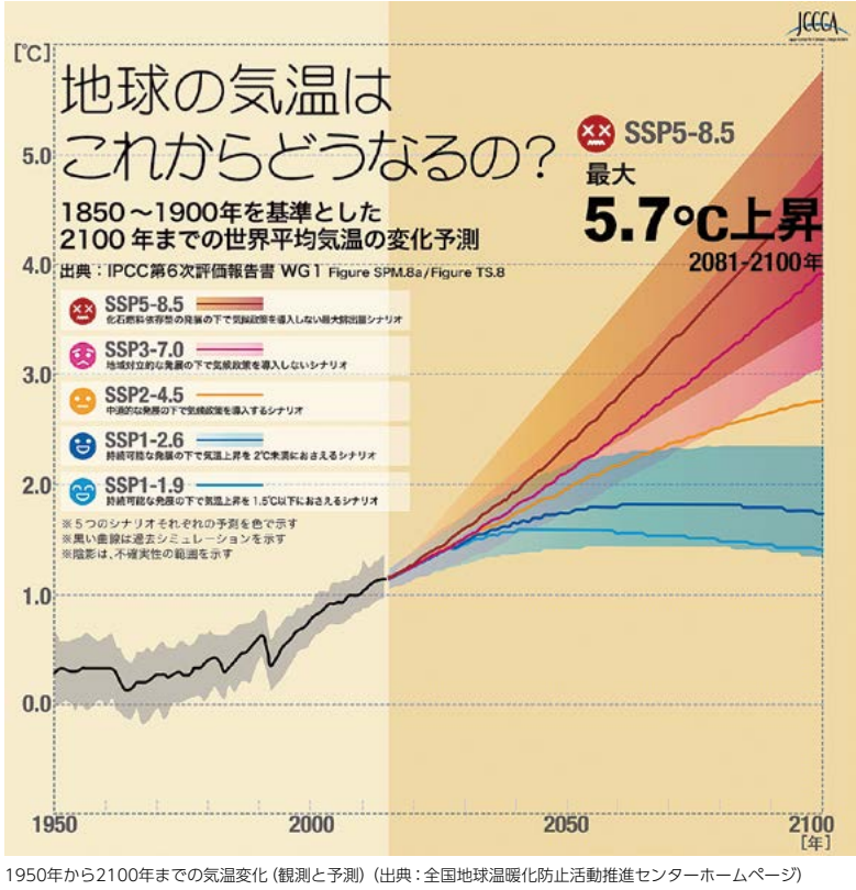
1950年から2100年までの気温変化(観測と予測)(出典: 全国地球温暖化防止活動推進センターホームページ)
