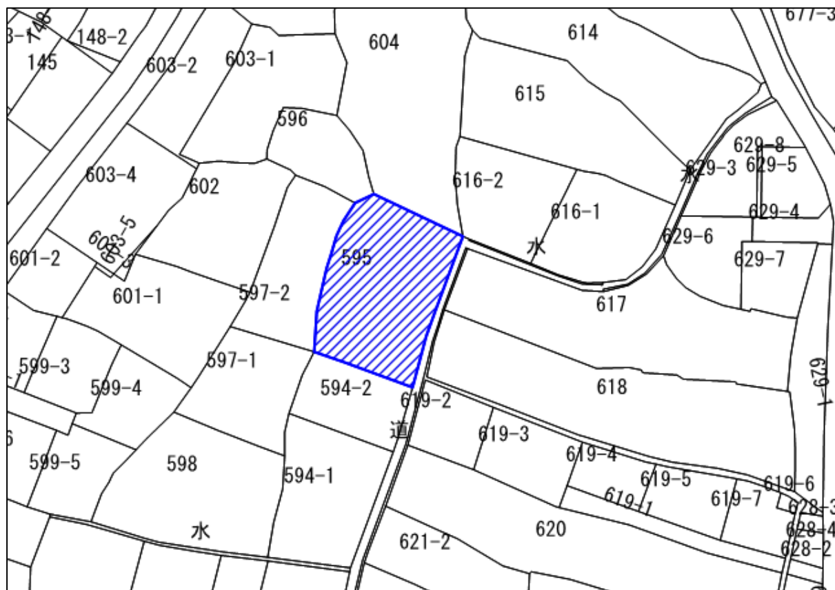
地籍図
