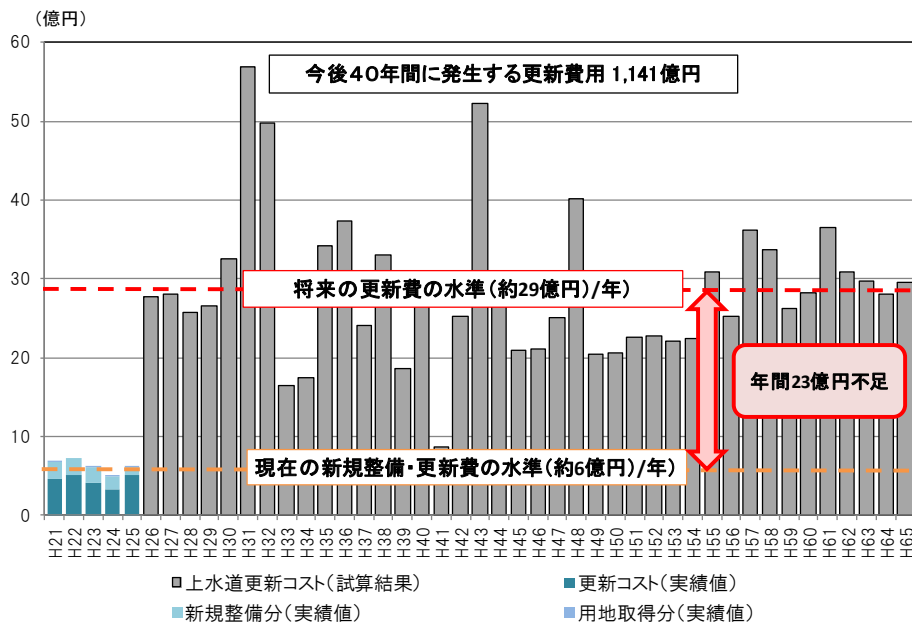
図表 19 水道施設の今後の更新コスト
