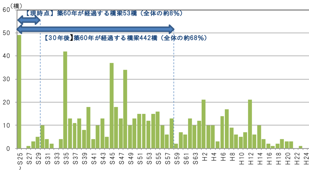
図表 15 橋梁の年度別整備状況
