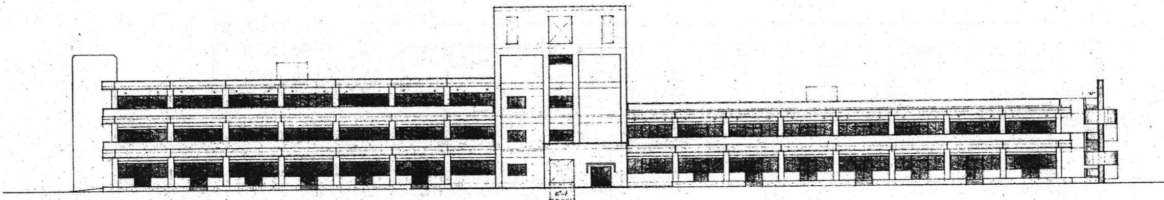
北側立面図
