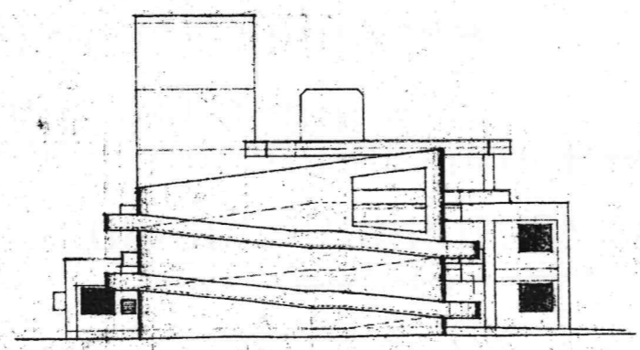
西側立面図
