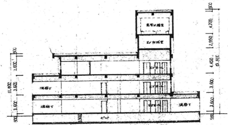
断面図
